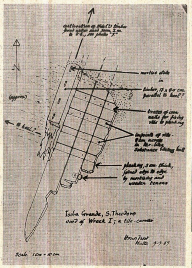
Il rilievo in scala del relitto della nave romana compiuto dal sommozzatore archeologico inglese Miss Honor Frost
