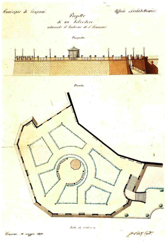
Progetto della costruzione di un belvedere sul bastione di San Francesco D'Assisi anno 1871
